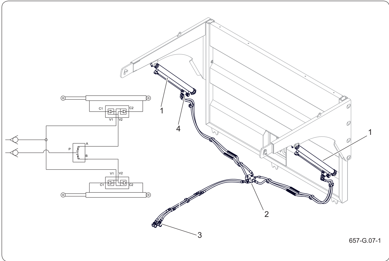
Figure 4.6 Construction et schéma du circuit hydraulique du hayon
