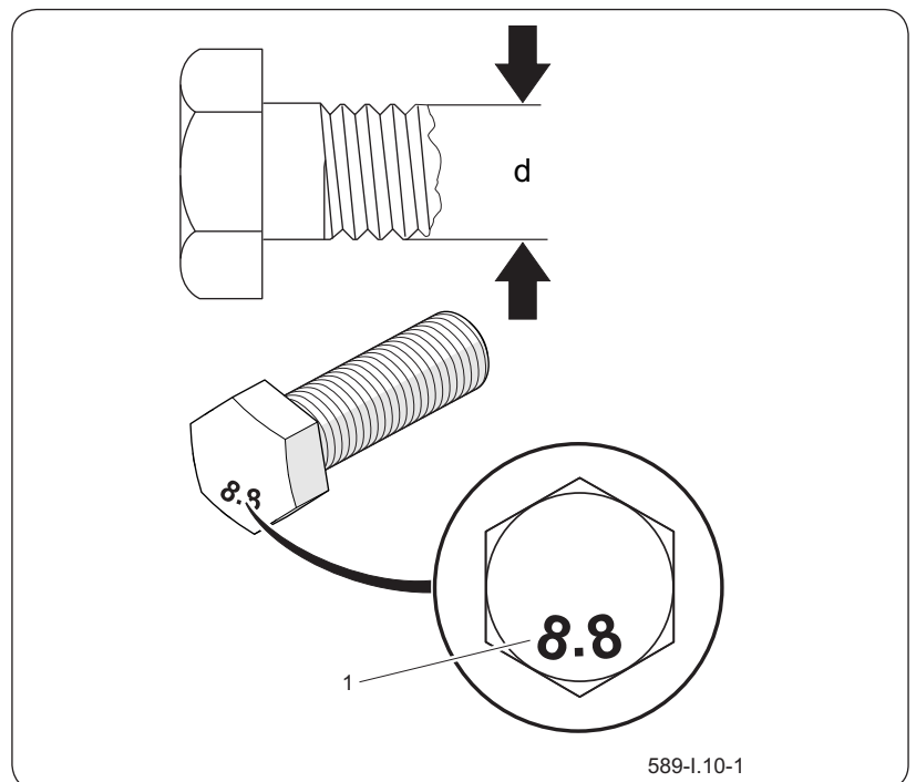
Figure 6.22 Vis avec filetage métrique (1) classe de résistance, (d) diamètre de filetage
