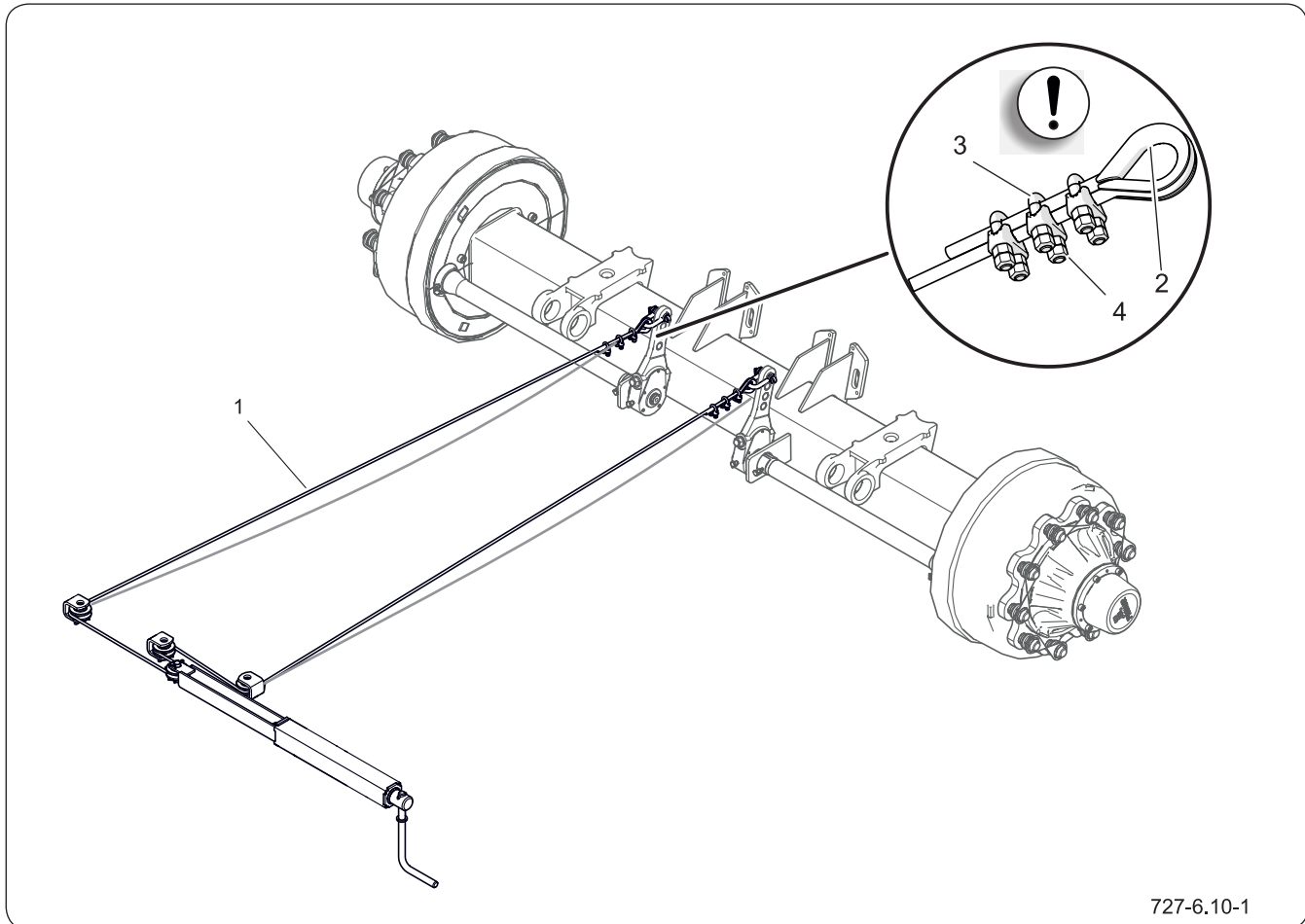
Figure 6.20 Remplacement du câble du frein de stationnement
