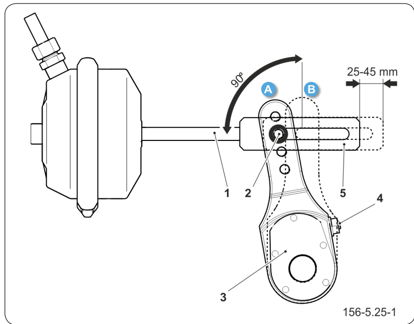
Figure 6.18 Réglage du frein
