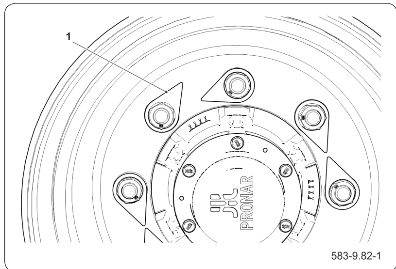
Figure 6.14 Indicateurs de serrage
