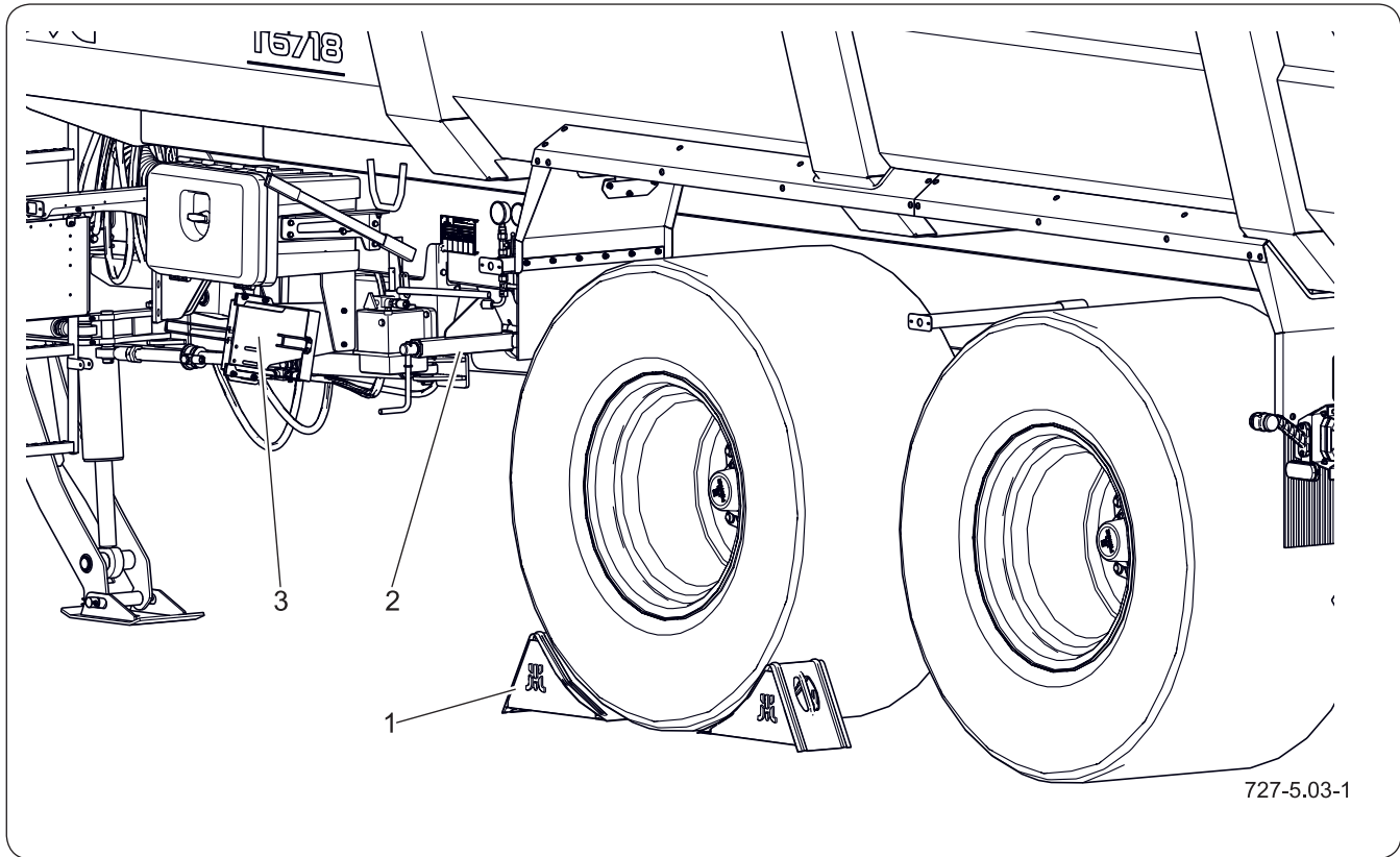
Figure 5.11 Frein de stationnement
