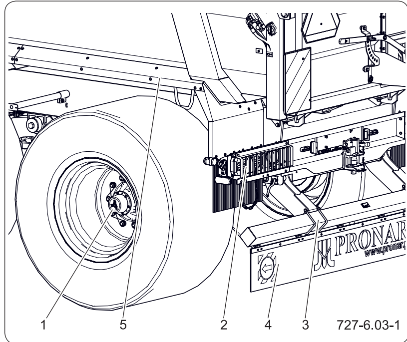
Figure 6.5 Capots de protection de la remorque (1) enjoliveur d'essieu (2) cache-feu (3) pare-chocs (4) bavette (5) déflecteurs
