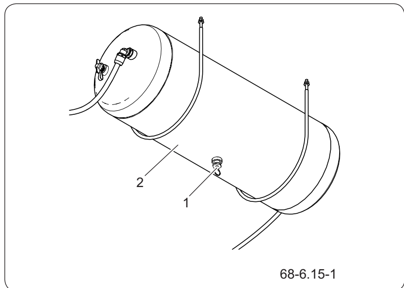
Figure 6.6 Réservoir d'air
