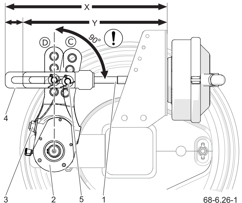
Figure 6.16 Contrôle du frein
