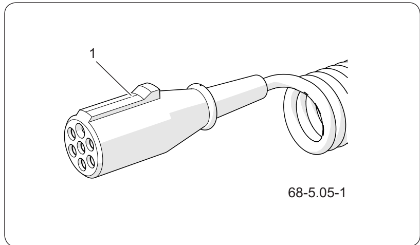
Figure 5.15 Raccordements de l'installation électrique
