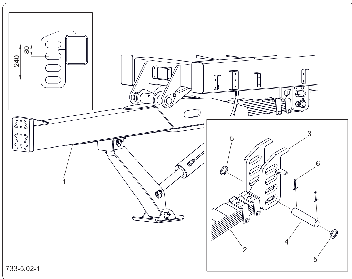
Figure 6.1 Amortissement mécanique du timon
