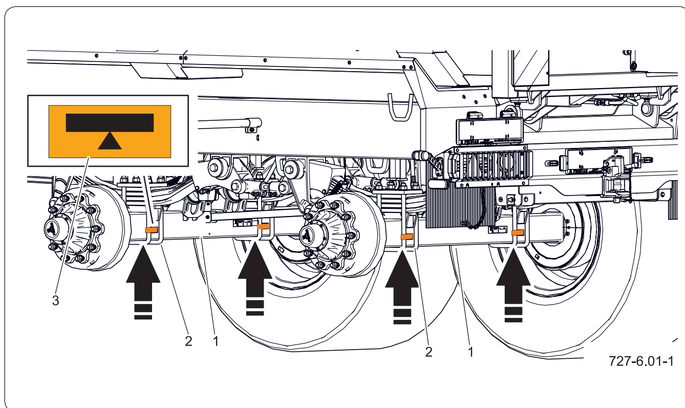
Figure 6.2 Points d'appui recommandés pour la remorque
