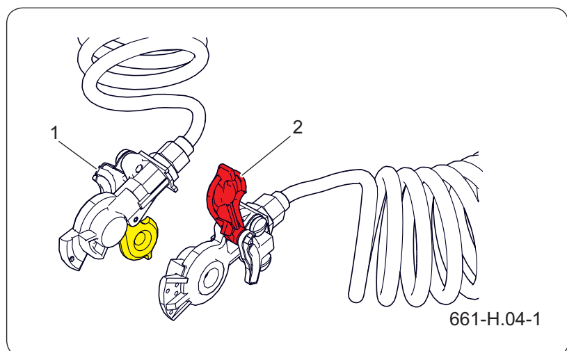
Figure 5.13 Conduites du système de freinage pneumatique
