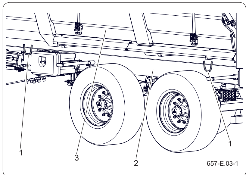
Figure 2.8 Points de fixation (1) poignée (2) châssis inférieur (2) benne
