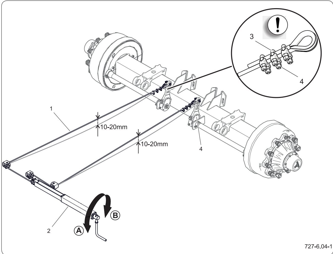
Figure 6.19 Vérification de la tension du câble
