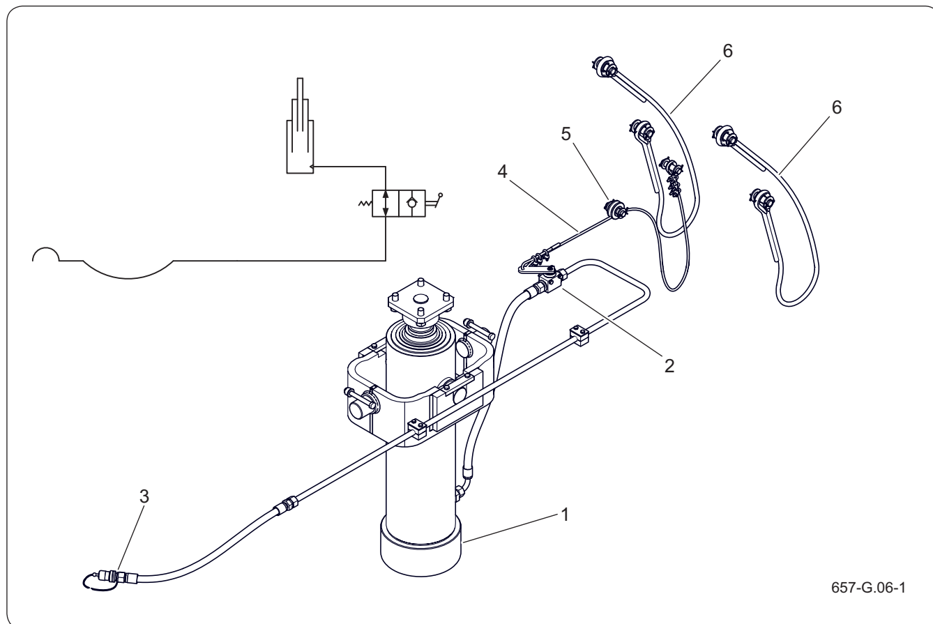
Figure 4.5 Construction et schéma de l'installation hydraulique du dispositif de basculement
