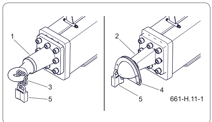
Figure 5.12 Protection du bras d'attelage
