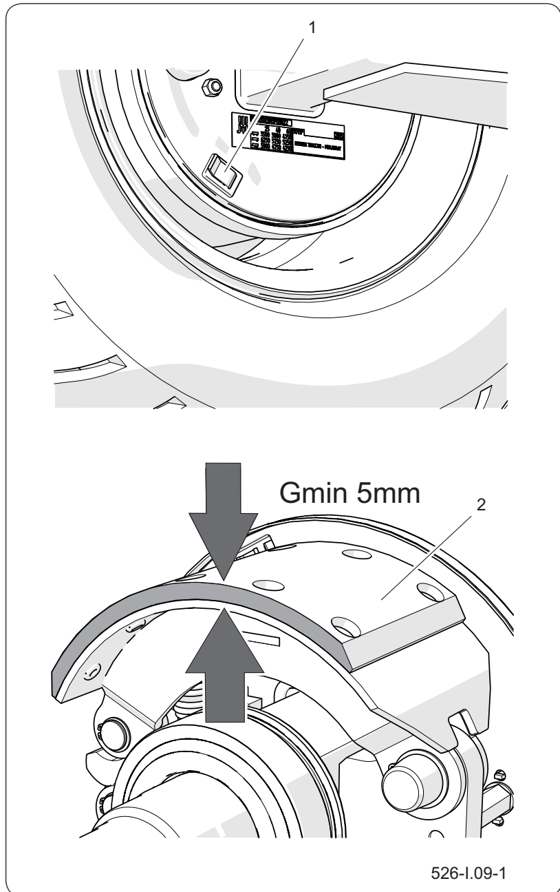
Figure 6.21 Contrôle de l'épaisseur des garnitures de frein
