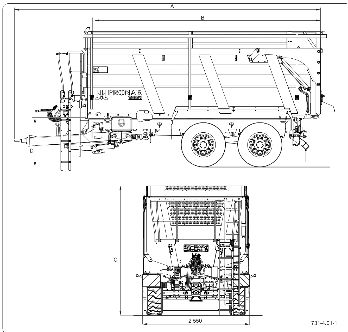
Figure 4.1 Dimensions de base de la remorque
