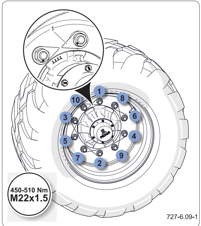
Figure 6.13 Ordre de serrage des écrous (1) indicateur de desserrage d'écrou
