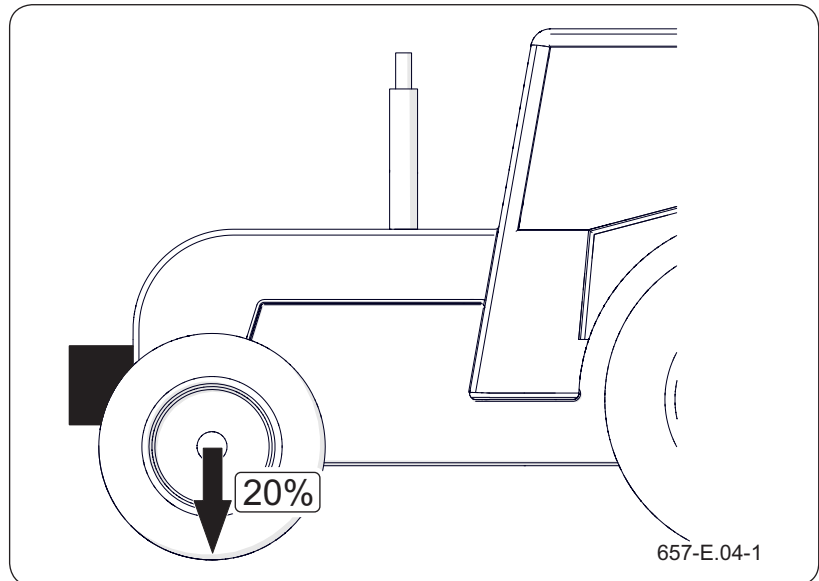
Figure 2.7 Charge minimale sur l'essieu avant du tracteur
