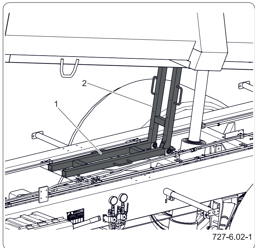
Figure 6.3 Béquille de la benne (1) béquille abaissée (2) béquille relevée
