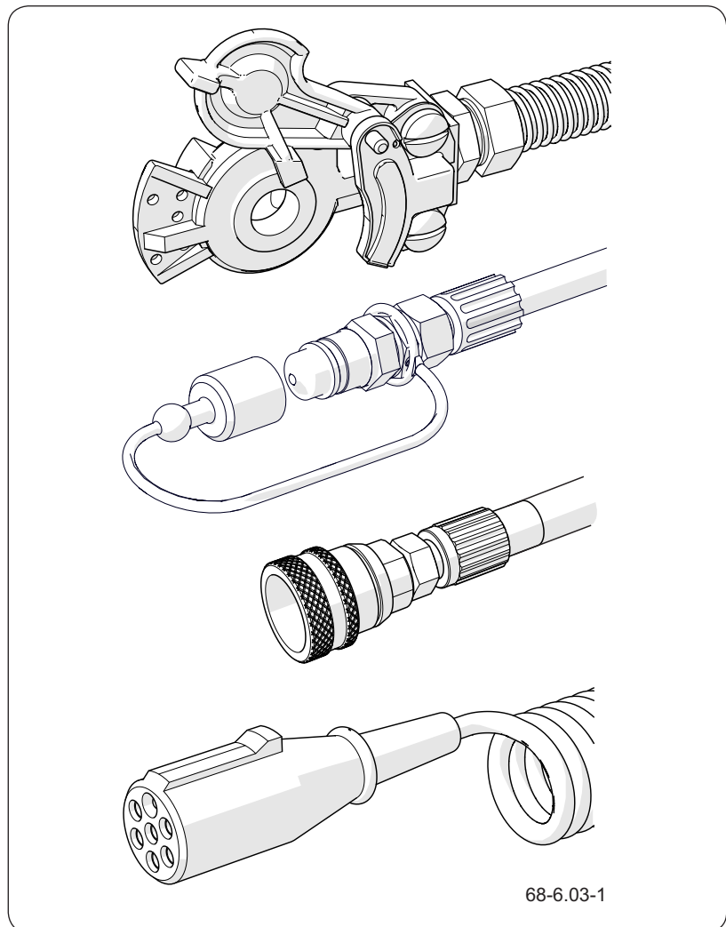
Figure 6.8 Coupleurs de la remorque (exemples)
