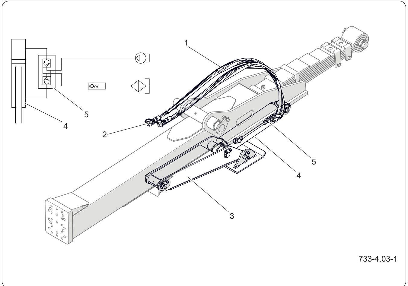
Figure 4.7 Construction et schéma de l'installation hydraulique de la béquille à ciseaux (1) conduit hydraulique (2) fiche hydraulique (3) béquille à ciseaux (4) actionneur hydraulique (5) verrou hydraulique
