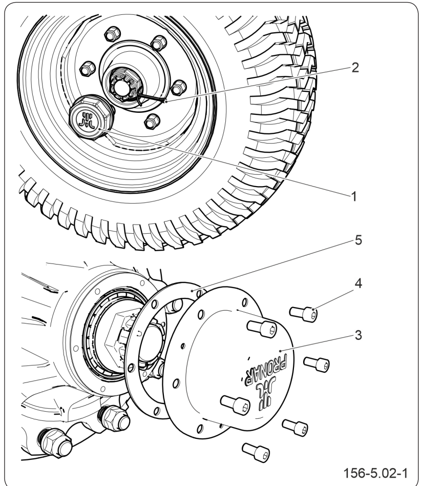
Figure 6.11 Démontage du couvercle et de la goupille
