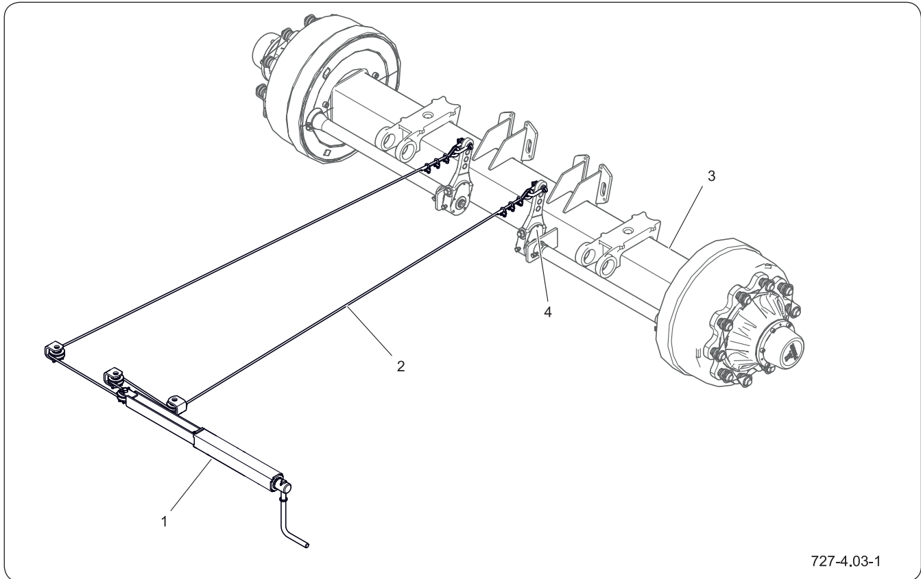
Figure 4.4 Construction du frein de stationnement
