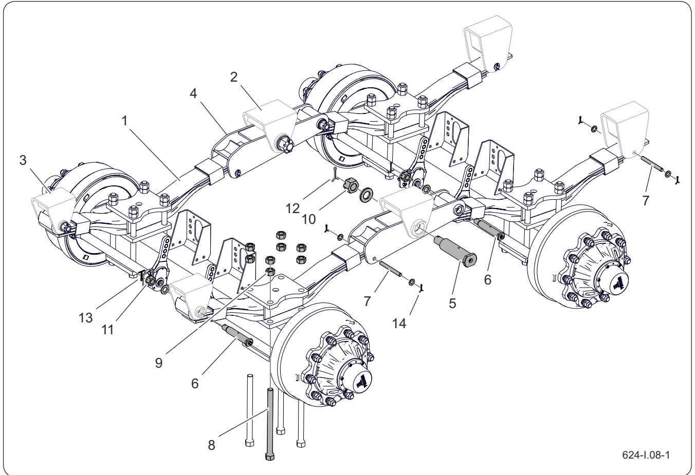
Figure 6.23 Entretien de la suspension mécanique
