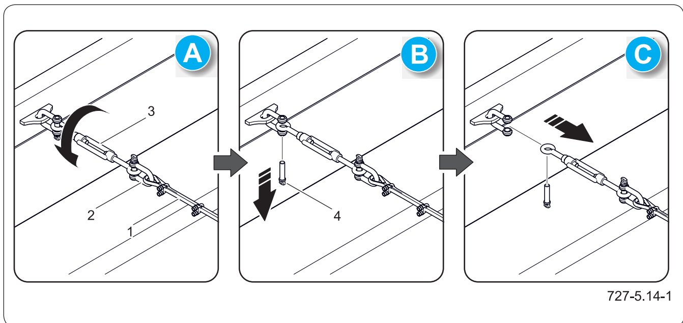
Figure 5.20 Câble de liaison
