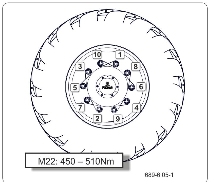
Figure 6.12 Ordre de serrage des écrous
