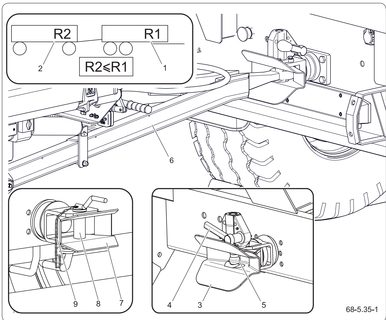
Figure 5.22 Agrégation de la seconde remorque
