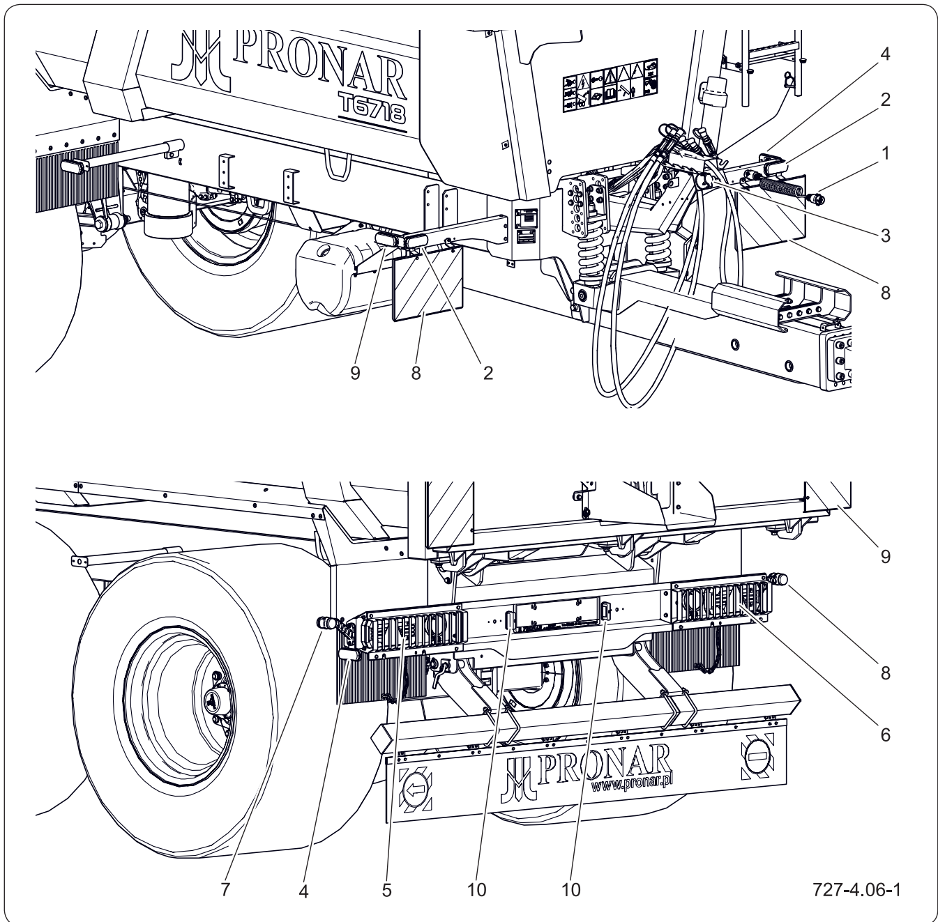
Figure 4.10 Disposition des éléments de l'installation électrique et des dispositifs réfléchissants – rampe d'éclairage complète.
